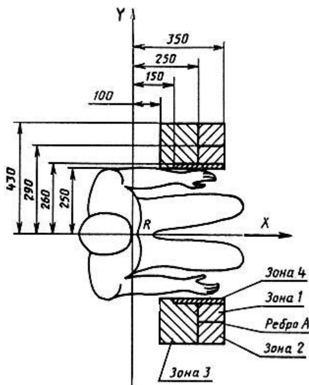
Чертеж. Расположение приводных элементов кнопочного управления краном
